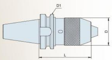
BT Shank JIS B 6339(MAS 403 BT)
